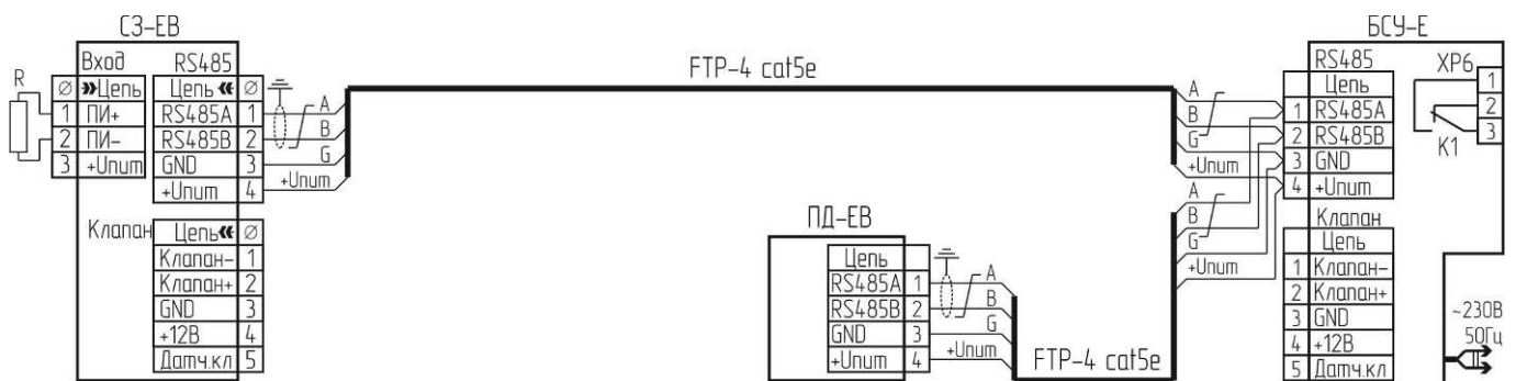
R – резистор типа C2-33-4,3кОм-20% (входит в комплект поставки сигнализатора) Подключение пожарных извещателей условно не показано.
