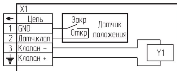
Рисунок 5 – Клапан КЗГЭМ-У. Схема электрическая принципиальная.
